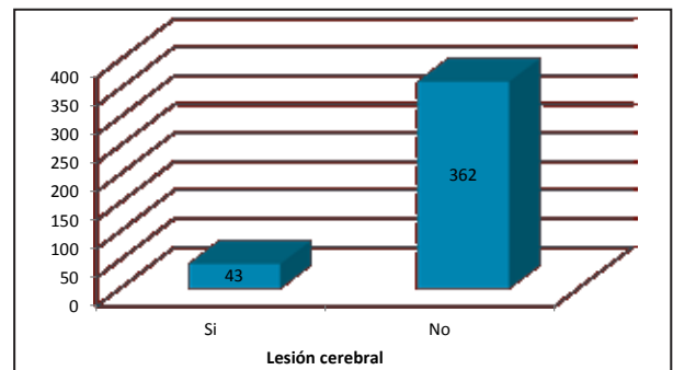
Figura 4. Evaluación neuropsicológica.
